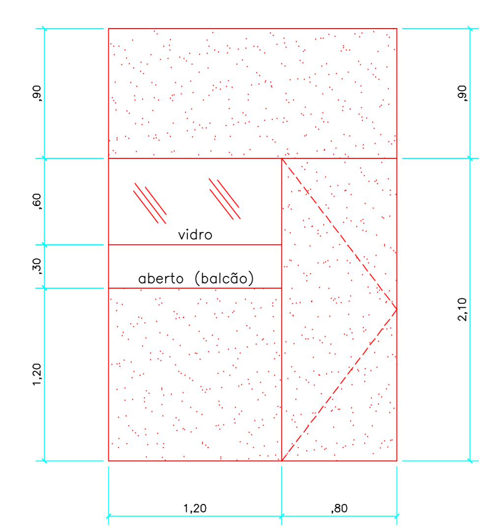
DETALHE 1 - VISTA Guichê e porta ESCALA 1:25
